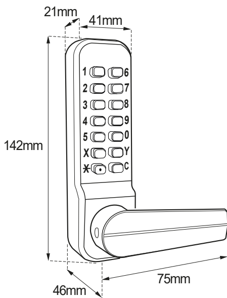
BL2400 ECP - Keypad
