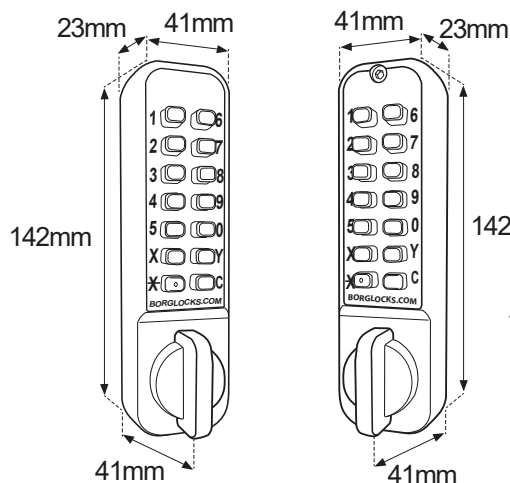
BL2127 ECP External Keypad
