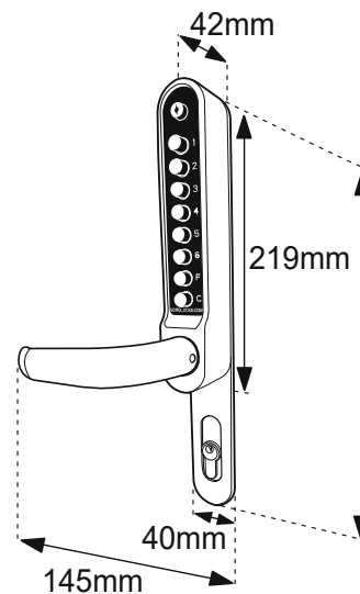
BL6100 ECP - Keypad
