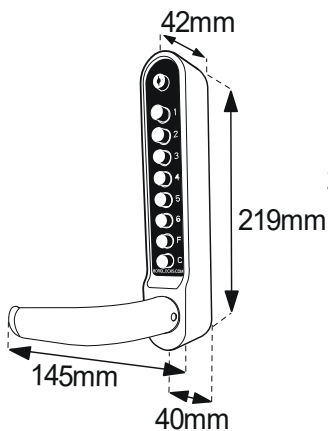
BL6000 ECP - Keypad
