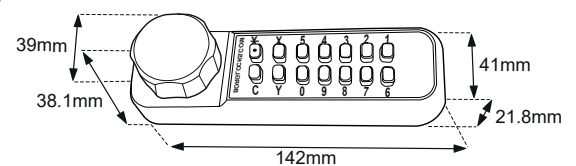
BL2615 ECP Keypad
