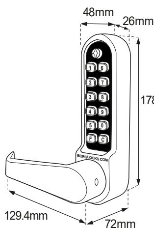
BL5400 ECP - Keypad
