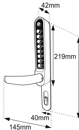
BL6100 ECP - Keypad
