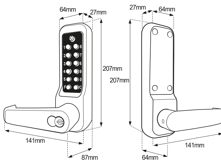
BL7700 ECP Keypad
