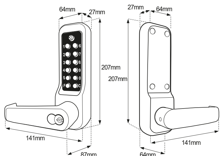
BL7700 ECP Keypad
