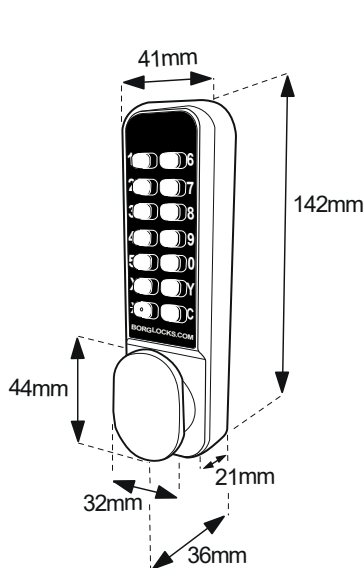
BL2000 ECP - Keypad
