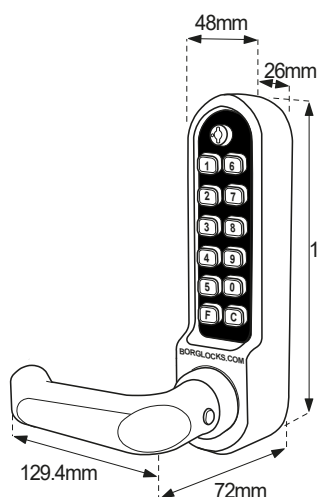
BL5000 ECP Keypad
