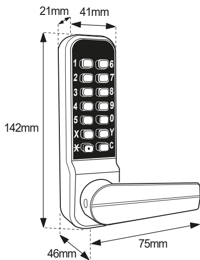
BL2400 ECP - Keypad
