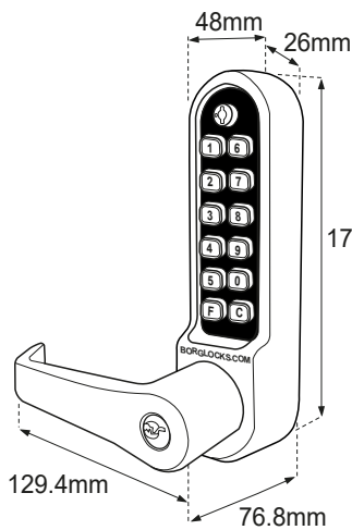
BL5700 ECP - Keypad
