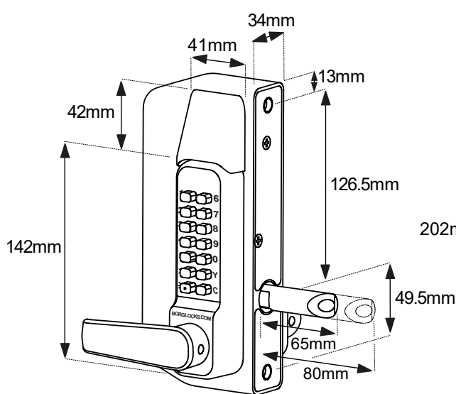
BL3400 ECP Keypad
