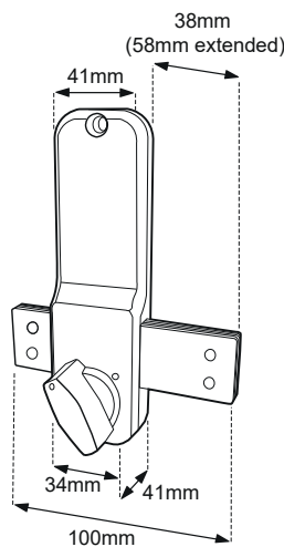
BL2605 ECP Deadbolt
