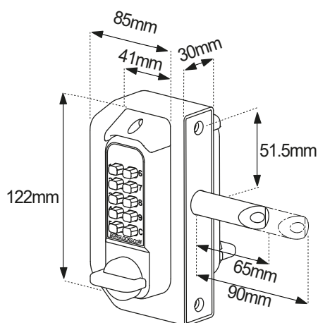
BL3030 ECP Keypad
