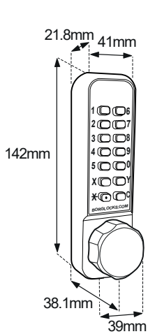
BL2600 ECP Keypad
