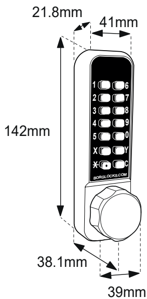
BL2500 ECP - Keypad
