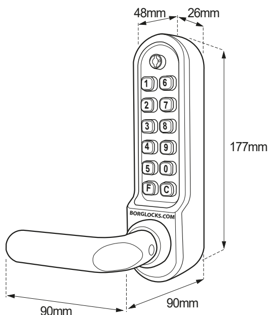
BL5200 ECP - External keypad
